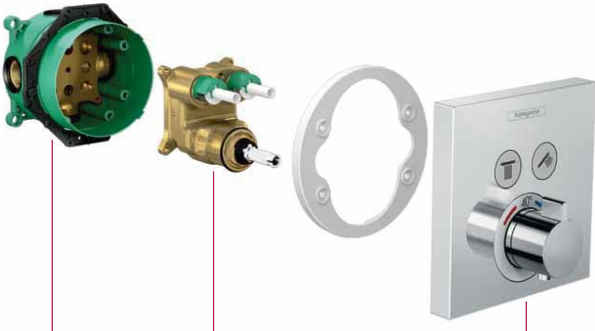
iBox® universal runko-osa
