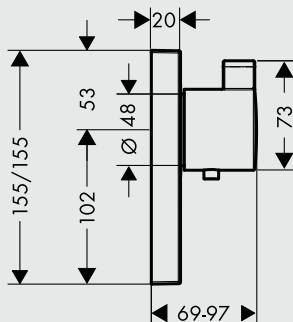
ShowerSelect® ShowerSelect-termostaatti Highflow yhdele suihkulle (alla) ja lisäsuih- kulle (yllä) # 15761, -000
